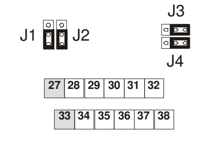
Рис. 4: расположение переключек на модуле DE200 V
